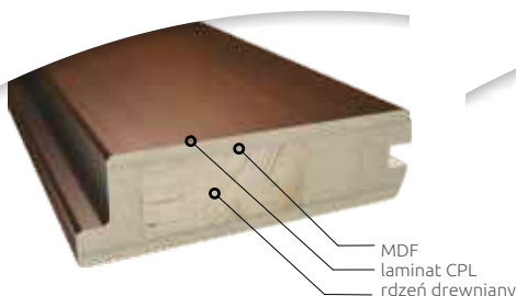
Ramiak konstrukcyjny typ 1
