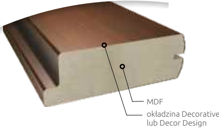
Ramiak konstrukcyjny typ 3
