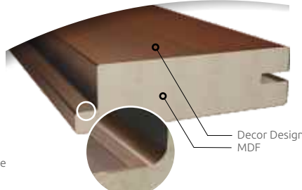
Ramiak konstrukcyjny typ 5
