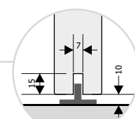
wręg na prowadnik
