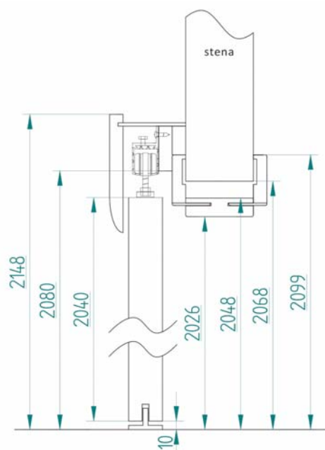
nástenný posuvný systém so zabudovaním
