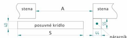
posuvný nástenný systém bez zabudovania
