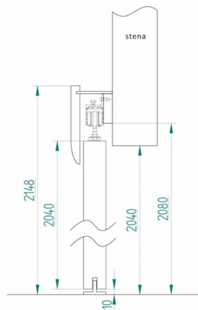
posuvný nástenný systém bez zabudovania
