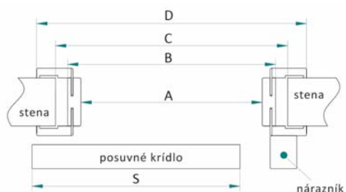
nástenný posuvný systém so zabudovaním
