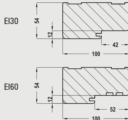
Przekrój ościeżnicy drewnianej p.poż do skrzydeł OLIMP
