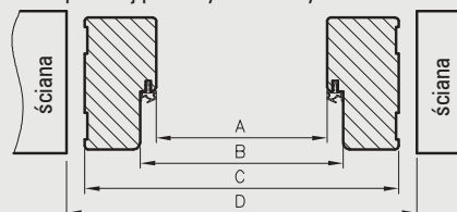
przekrój poziomy ościeznicy w murze
