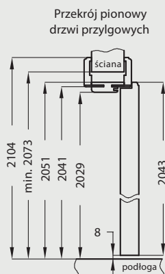
wymagana wysokość otworu w murze 2073 mm
