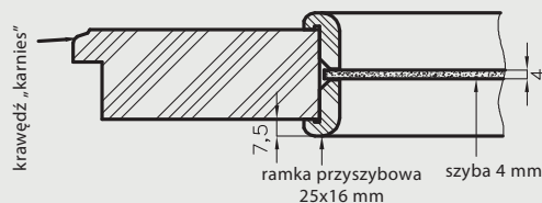
konstrukcja skrzydeł bezprzylgowych TOP (nie dotyczy kolekcji Carla TOP i Aldea TOP)
