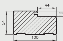
przekrój poziomy ościeznicy w murze
