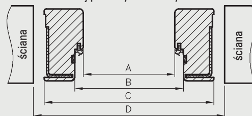
Przekrój poziomy ościeżnicy w murze
