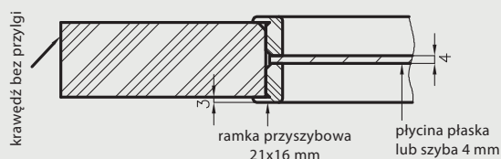
Konstrukcja skrzydeł przylgowych Natura
