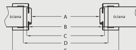
D - wymagana szerokość otworu w murze
