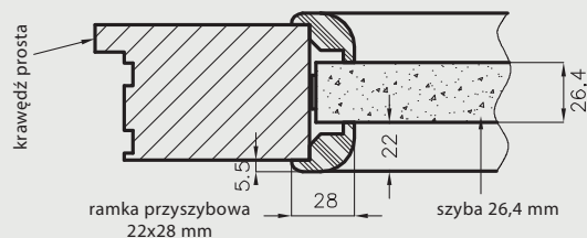
Konstrukcja skrzydeł przeciwpożarowych Olimp EI60
