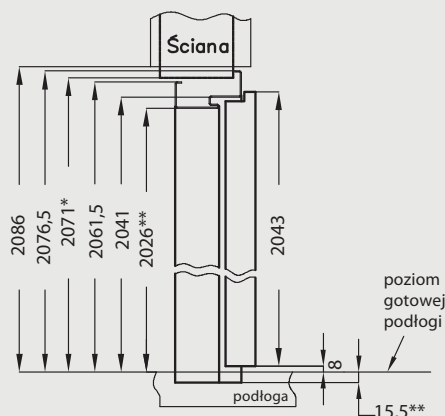
Przekrój pionowy
