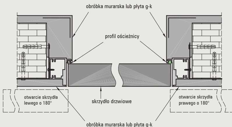
Przekrój poprzeczny drzwi Sara Eco
