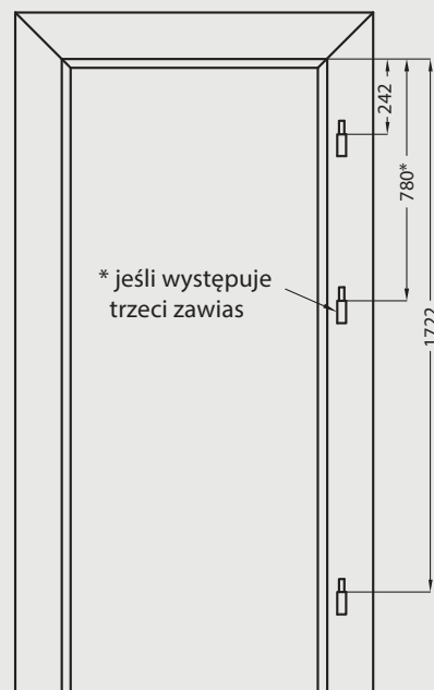
Przekrój poziomy
