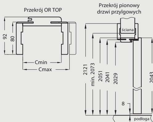
wymagana wysokość otworu w murze 2073 mm
