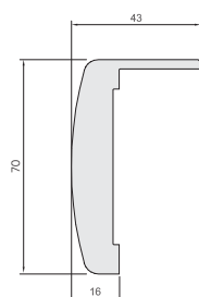
Element narożny ościeżnicy LUX kątownik standard
