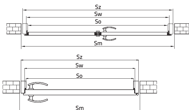
WYMIARY OŚCIEŻNIC STAŁYCH MU/U DO DRZWI DWUSKRZYDŁOWYCH W TECHNOLOGII STANDARD
