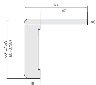
Element narożny ościeżnicy SW kątownik WYDŁUŻONY o 2cm
