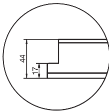
Przekrój skrzydła A2 32dB
