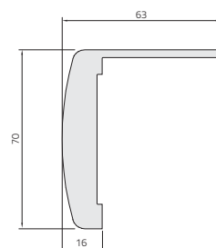
Element narożny ościeżnicy LUX kątownik WYDŁUŻONY o 2cm
