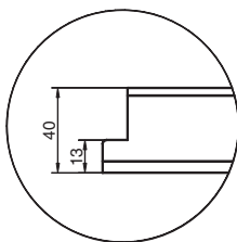
Przekrój skrzydła A1 30dB
