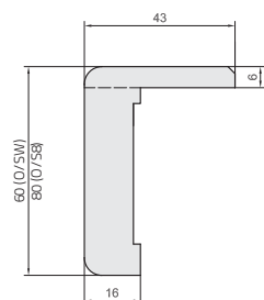
Element narożny ościeżnicy SW kątownik standard
