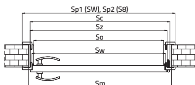
WYMIARY OŚCIEŻNIC REGULOWANYCH SW DO DRZWI DWUSKRZYDŁOWYCH W TECHNOLOGII STANDARD, SOFT ORAZ TECHNOLOGII RAMA SOFT WYMIARY STANDARDOWE
