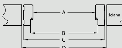
Przekrój poziomy
