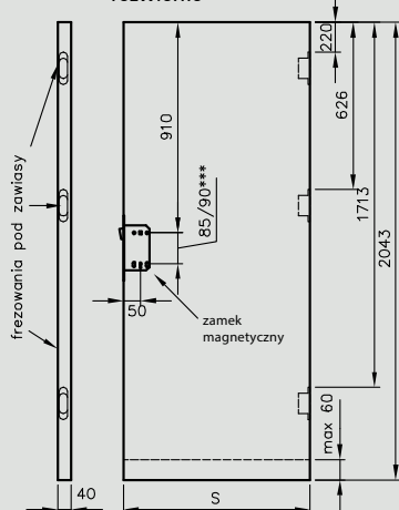
Skrzydła bezprzylgowe rozwiernie
