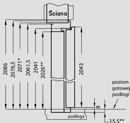
Przekrój pionowy
