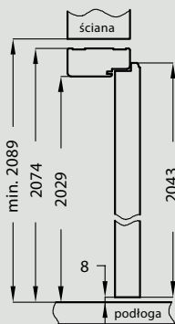
Przekrój pionowy drzwi przylgowych
