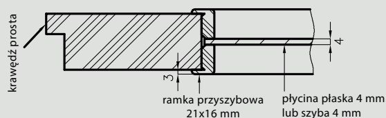
Konstrukcja skrzydeł Lack (nie dotyczy Lack 20s i 30s) i Ascada
