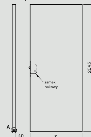
Skrzydła bezprzylgowe przesuwne
