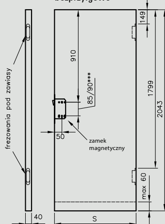
Skrzydła Sara Eco bezprzylgowe
