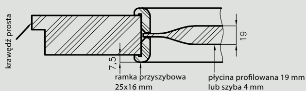
Konstrukcja skrzydeł przeciwpożarowych Olimp EI30
