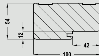
Przekrój ościeżnicy drewnianej p.poż do skrzydeł OLIMP
