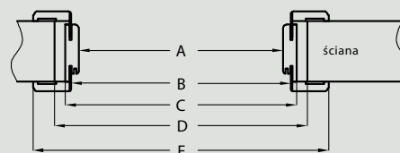
Przekrój poziomy
