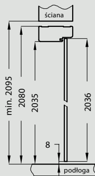
Przekrój pionowy drzwi szklanych
