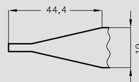
profil płyciny MDF 19 mm (Scala B, Trevi, Piano 9-12, Elsa, Nestor)
