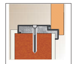
Montaż na dyble.
