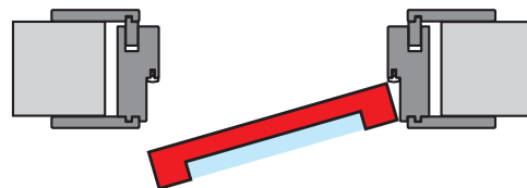
SPOSÓB MONTOWANIA SZYBY MATOWEJ (SKRZYDŁO PRAWY – CZĘŚĆ MATOWA OD STRONY OBSERWATORA)
