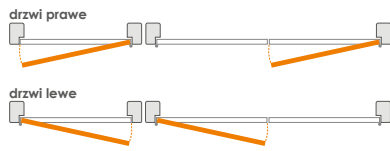
WYMIARY SKRZYDEŁ PRZYLGOWYCH
